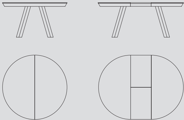
Ref. 5010 Ø125 (165x125) · Ø140 (185x140) · Ø150 (200x150)
