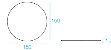
1345 Piano in gres per tavolo tondo 6/7 posti 6/7 seats gres round table top x cod. 1358 ø150 - H1,2 Kg 50,6
