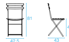
314 Sedia pieghevole Folding chair W42,5 - D43 - H81 Kg 4,8
