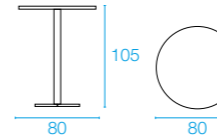
540 Tavolo alto tondo abbattibile 2/4 posti 2/4 seats collapsible round table ø80 - H105 Kg 15,7
